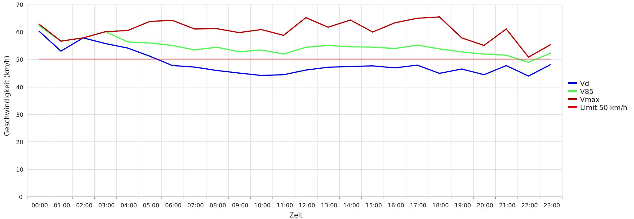
Biberen - Oberdorfstrasse 26, Fahrtrichtung Biberen, 50 km/h Beschränkung Vd, V85, Vmax vs. Uhrzeit
