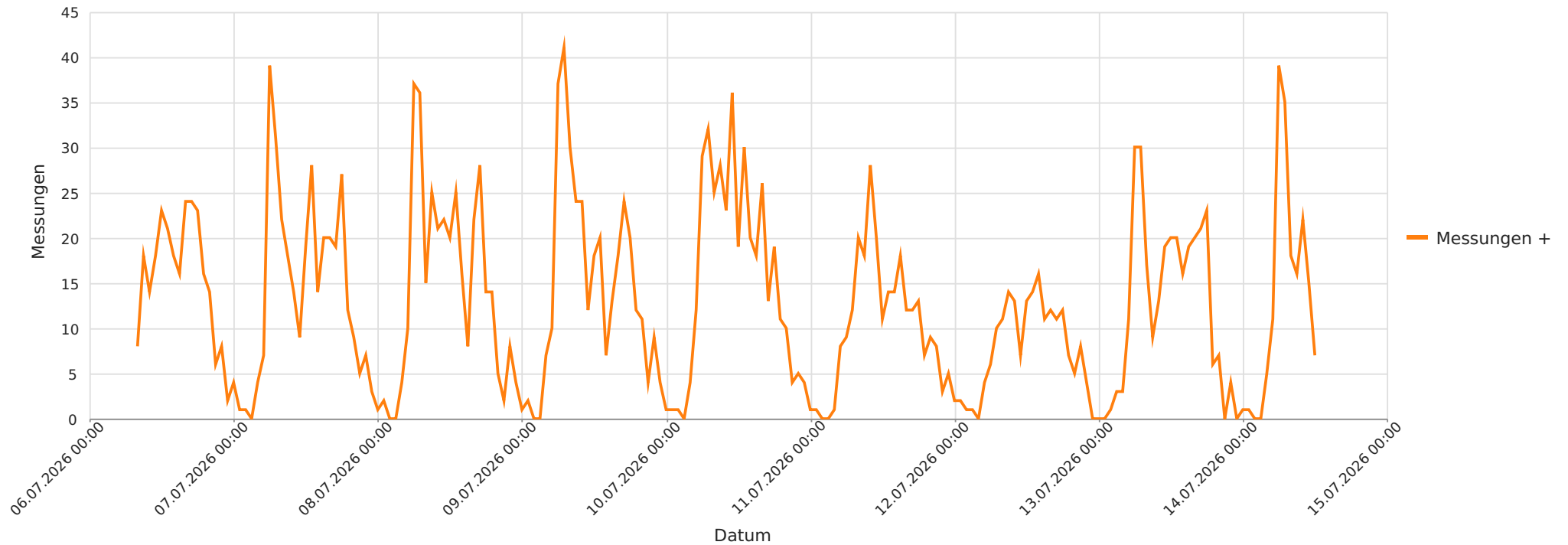
Biberen - Oberdorfstrasse 26, Fahrtrichtung Biberen, 50 km/h Beschränkung Anzahl der Messwerte vs. Messzeitraum
