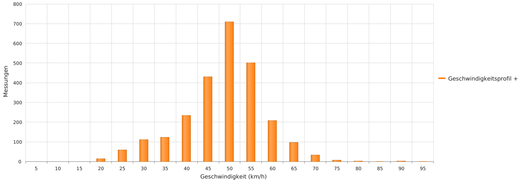
Biberen - Oberdorfstrasse 26, Fahrtrichtung Biberen, 50 km/h Beschränkung Anzahl der Messwerte vs. Geschwindigkeit
